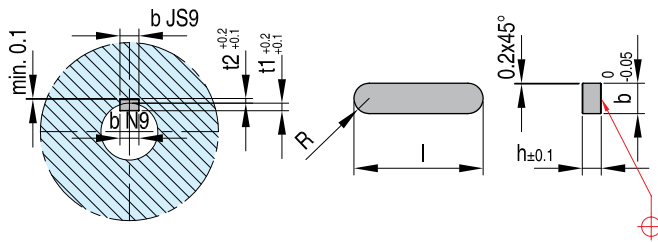
Установка сегментных шпонок
